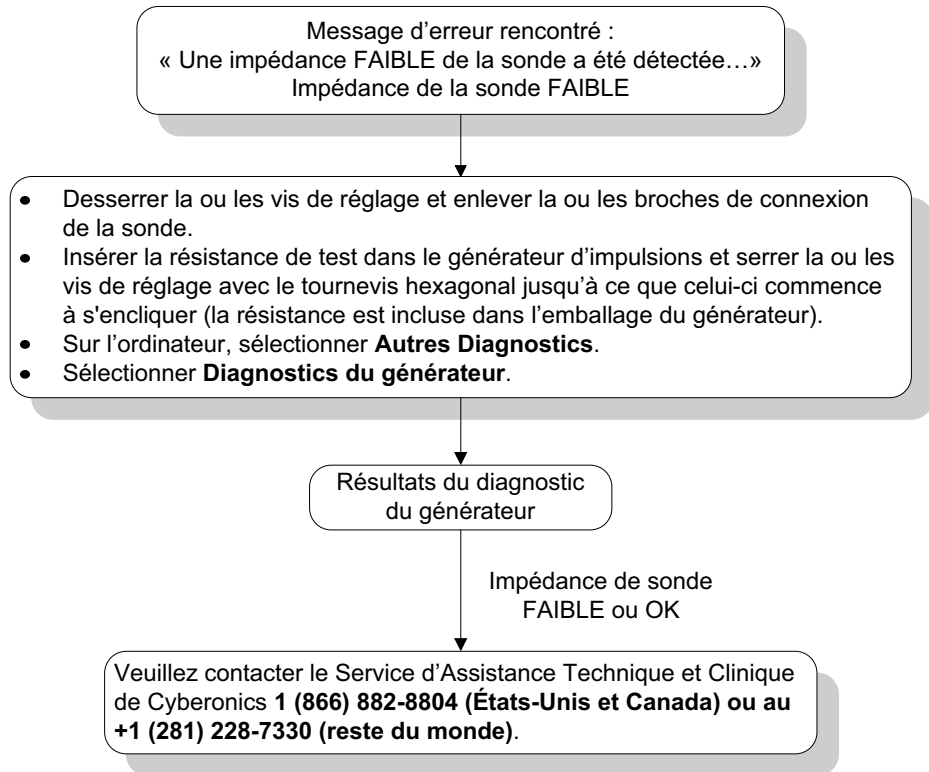
Figure 40. Impédance faible de la sonde pendant les diagnostics du système en salle d'opération—Remplacement du générateur d'impulsions
