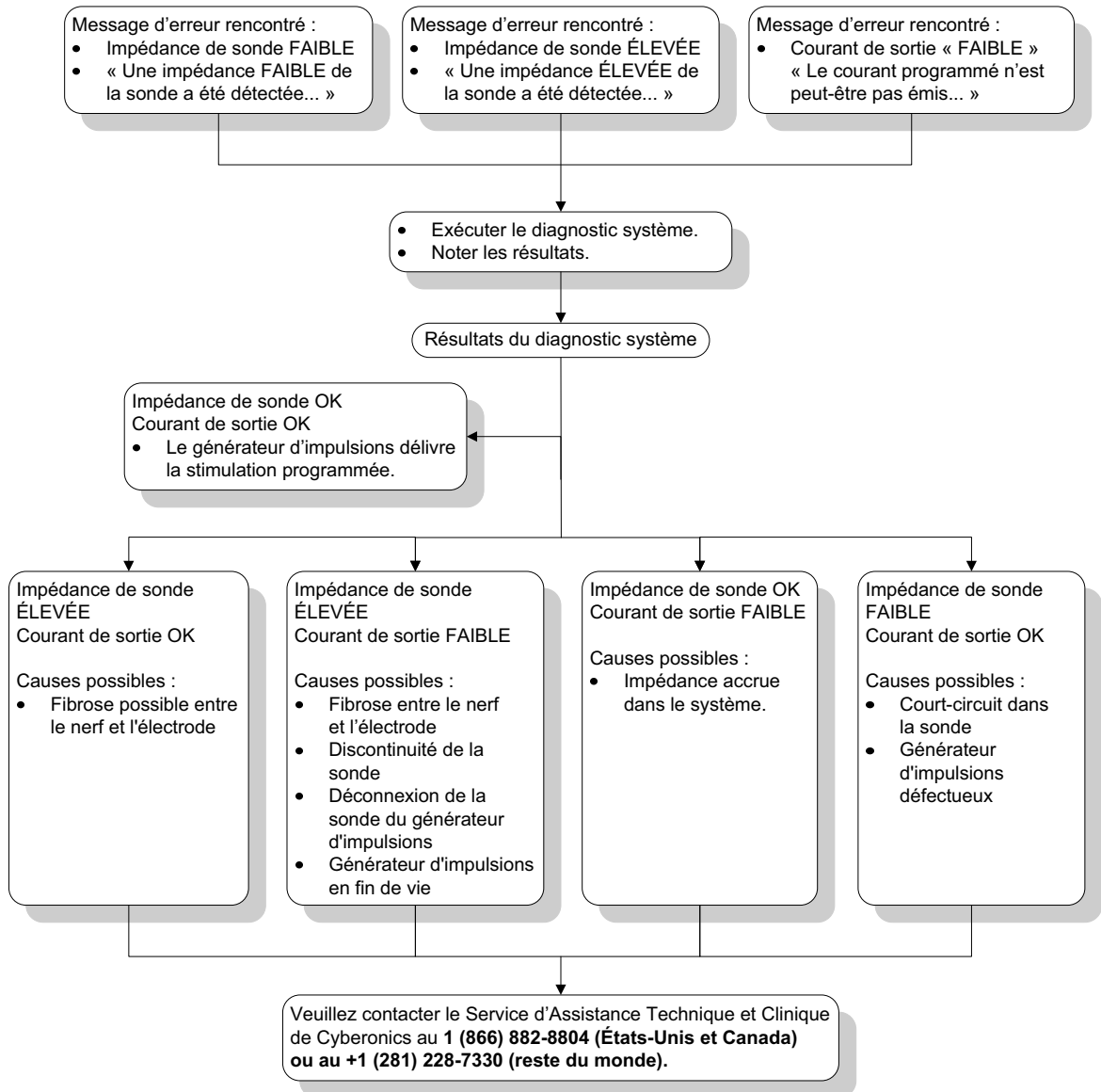
Figure 43. Le test de diagnostic ou une interrogation indiquent une impédance élevée de la sonde, une impédance faible de la sonde, ou un courant de sortie faible lors de la visite de suivi pour les générateurs d'impulsions modèles 103, 104 et 105
