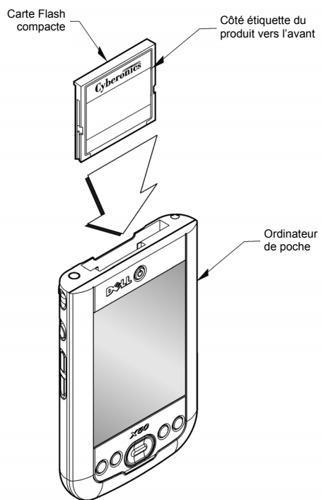
Figure 36. Orientation correcte de la carte Flash
