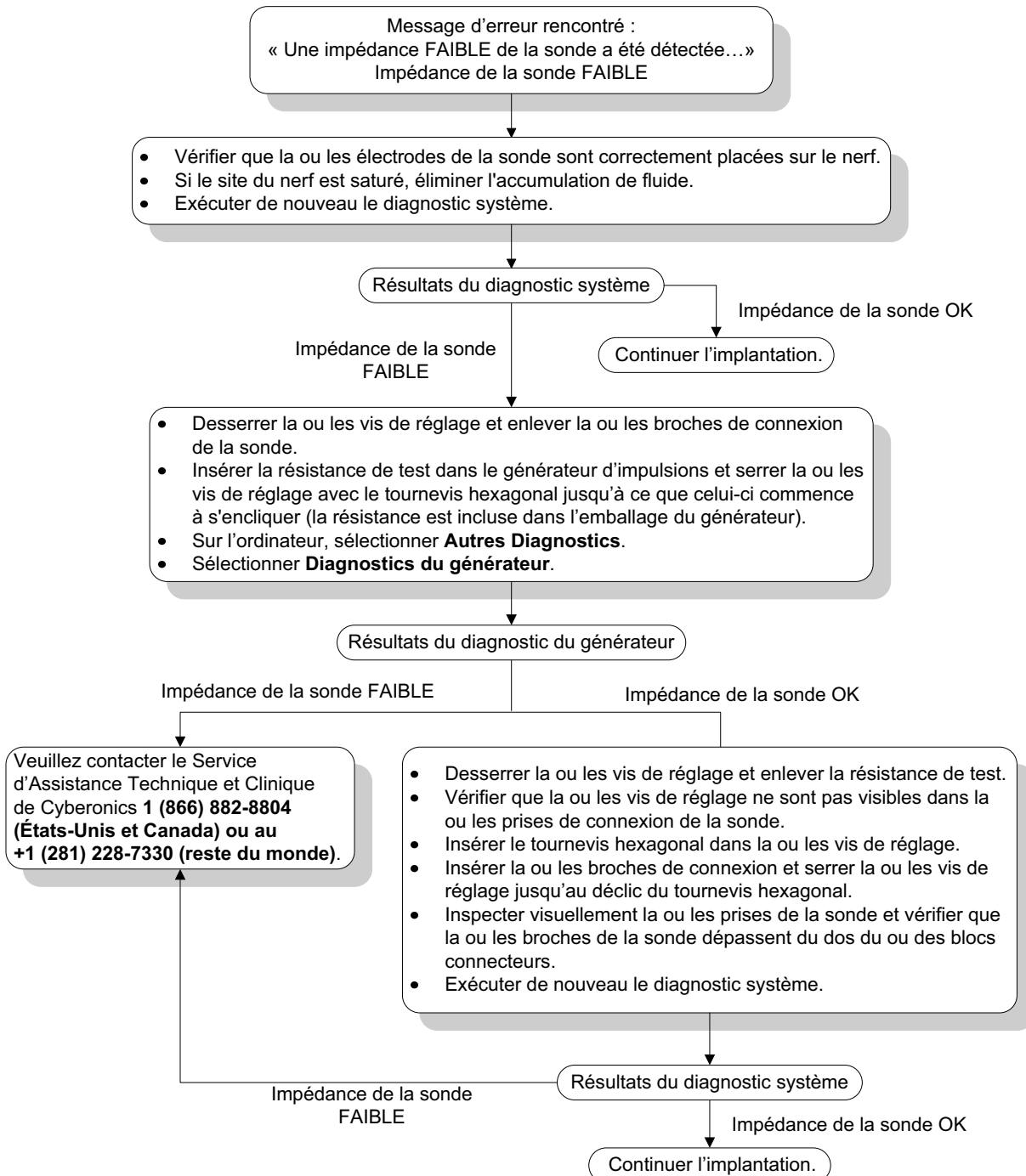
Figure 39. Impédance faible de la sonde pendant le diagnostic système en salle d’opération— Implant initial
