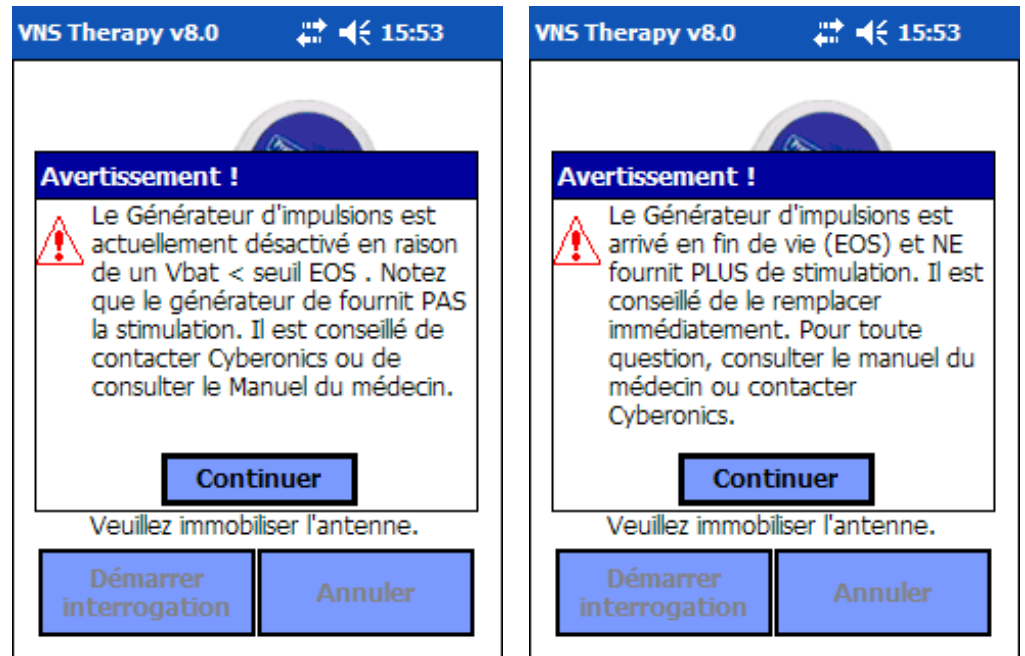
Figure 9. INDICATEUR D'ÉTAT DE LA BATTERIE et d'IMPULSION DESACTIVEE— Écran d'avertissement EOS
