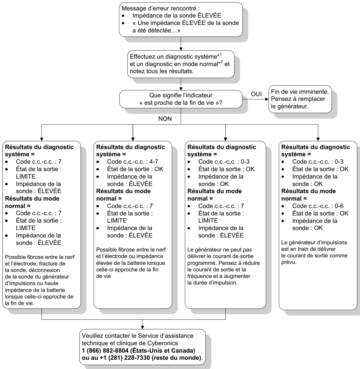
Figure 42. Le test de diagnostic indique une impédance élevée de la sonde lors de la visite de suivi pour les générateurs d'impulsions modèles 100, 101 et 102
