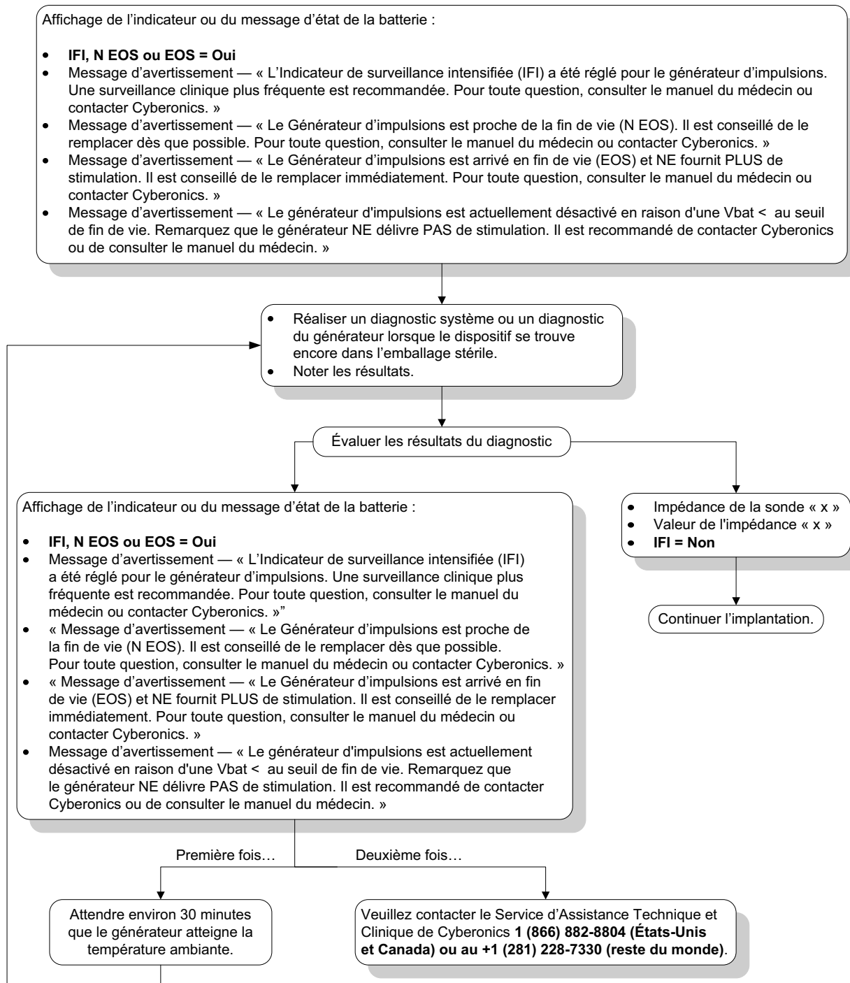
Figure 41. Indications de batterie faible/en fin de vie avant de procéder à la chirurgie hors du champ stérile—Implant initial ou remplacement du générateur d’impulsions
